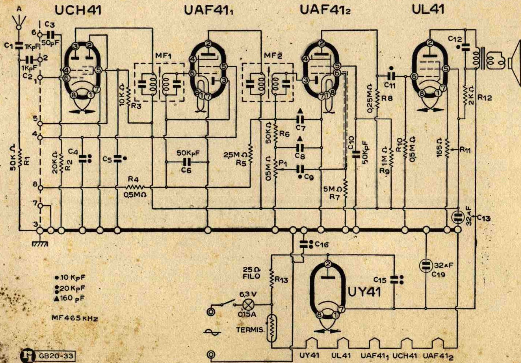
Lo schema elettrico del mod. D2
